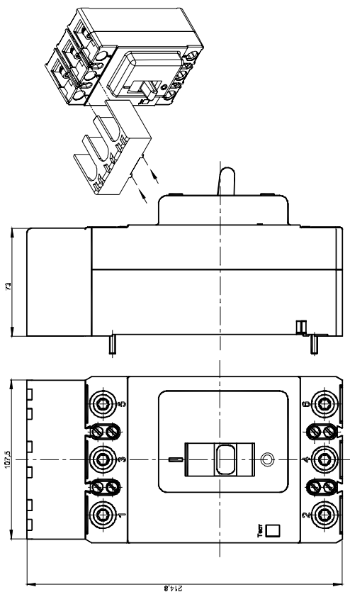
Рисунок Б.1 – Выключатель с ручным приводом: а) выключатель; б) выключатель с клеммной крышкой.
