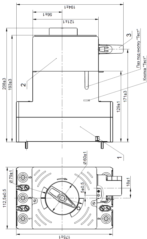
1 – выключатель; 2 – привод электромагнитный; 3 – соединитель типа РП10. Масса выключателя с электромагнитным приводом не более 4,1 кг.
