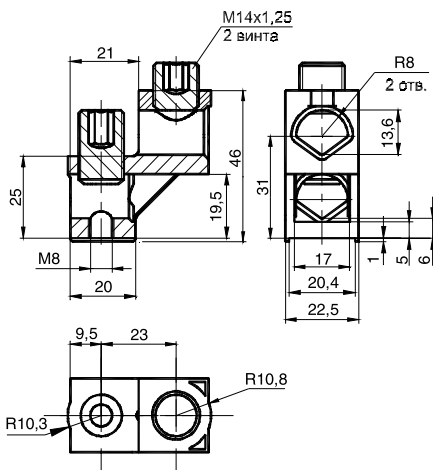
Двугнездный зажим для присоединения двух кабелей сечением до 95 мм 2
