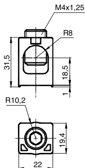
Одногнездный зажим для присоединения кабеля сечением до 185 мм 2
