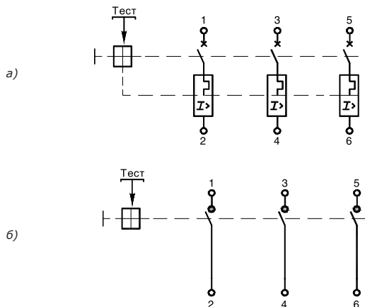
Рисунок В.1 – Схема электрическая принципиальная выключателя переменного тока трехполюсного исполнения: а) с тепловыми и электромагнитными расцепителями; б) без тепловых и электромагнитных расцепителей.
